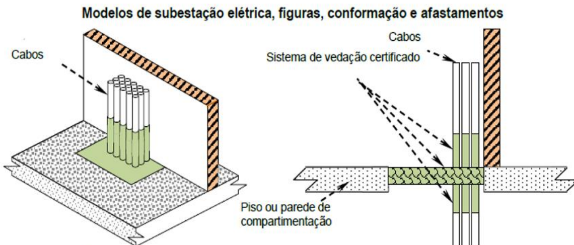
Figura A.1: Exemplo de vedação de abertura para passagem de cabos entre ambientes compartimentados
