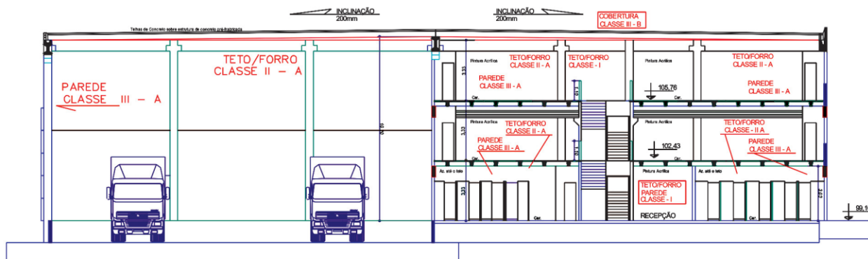
Corte AA
